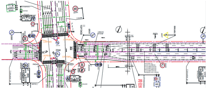
调整后车道布局
