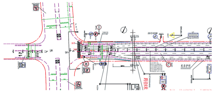
原车道布局
